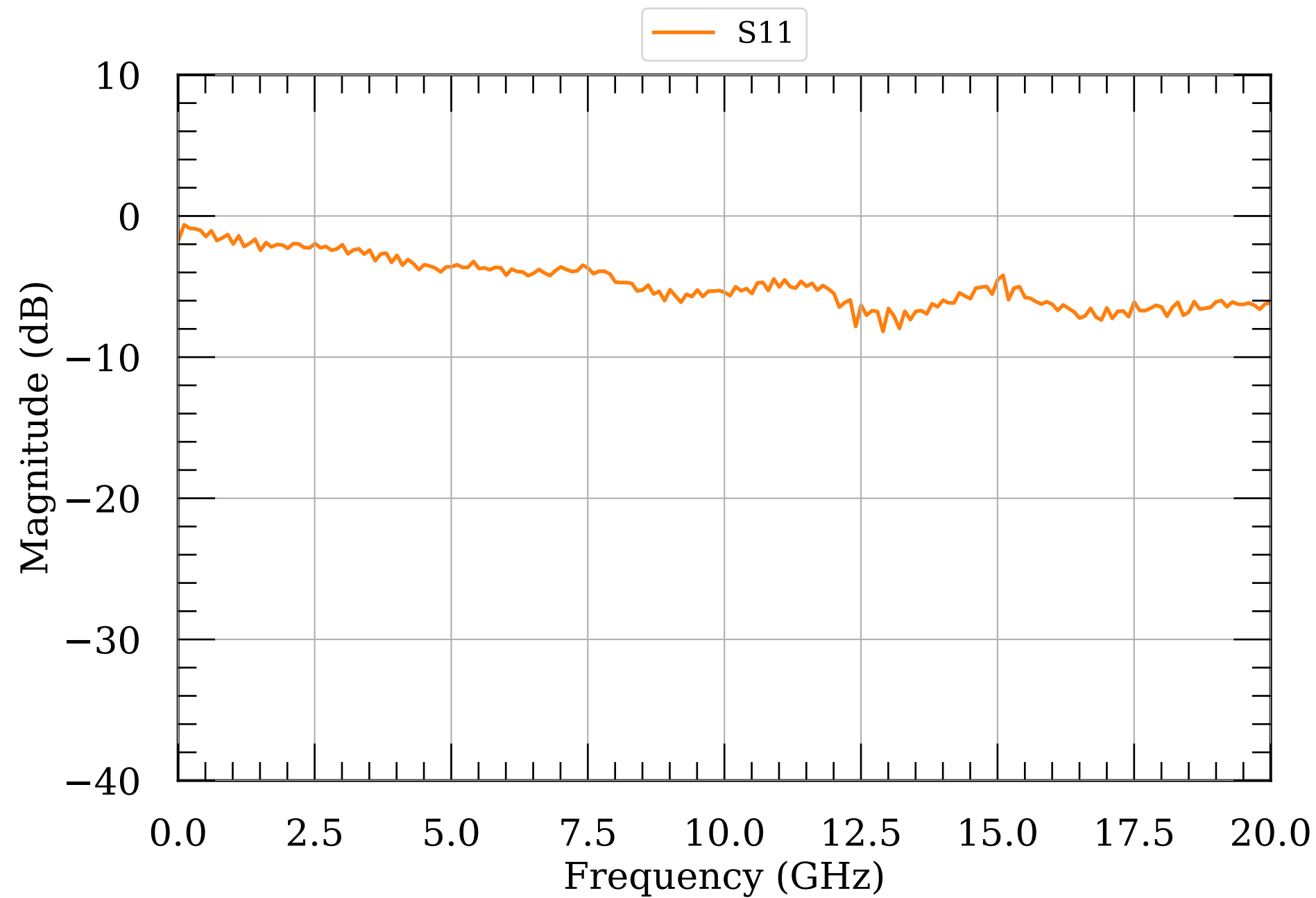
LNA S-params module019
